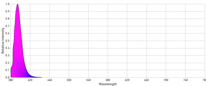
400nm | UVA
